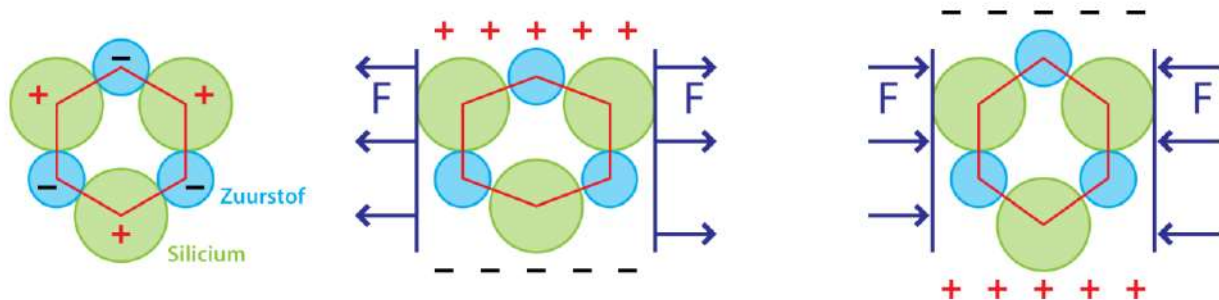
Figuur 22 Piëzo-elektrisch effect in kwarts ( \text{SiO}_2 ). Links: geen kracht, midden een trekkracht en rechts een duwkracht.
