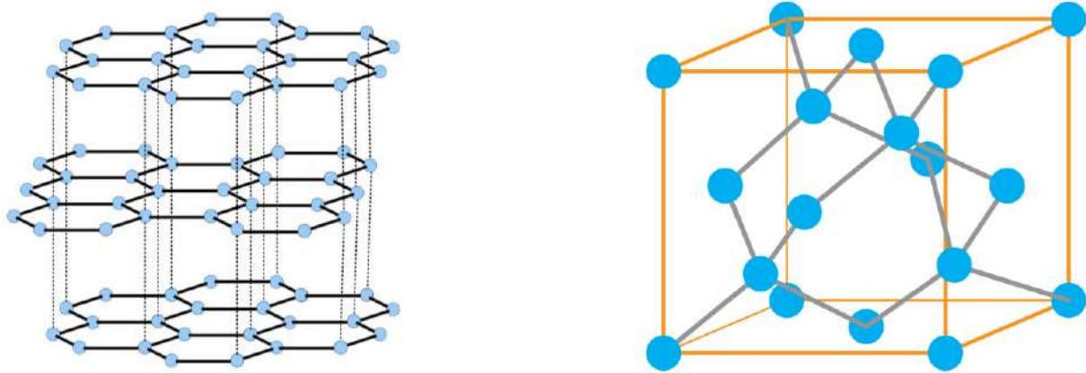
Figuur 29 Grafiet (links) en diamant (rechts).
