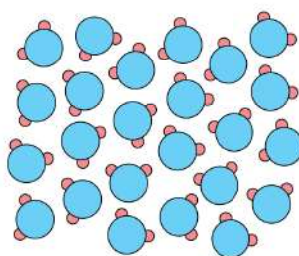
vloeibaar water
