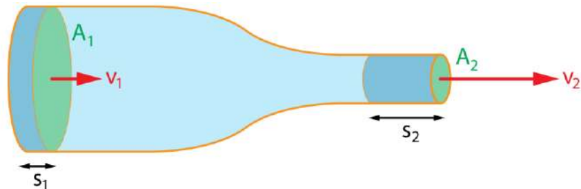
Figuur 16 Door ieder stukje pijp stroomt per seconde evenveel massa.
