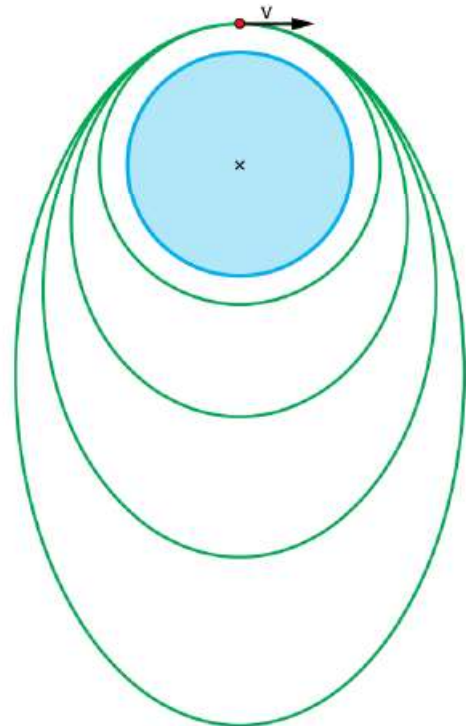
Figuur 33 Horizontaal weggeschoten projectiel met v_{\text{begin}} > 8,0 km/s.
