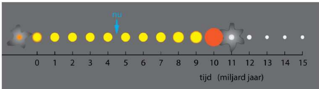
Figuur 64 De levensloop van de zon.
