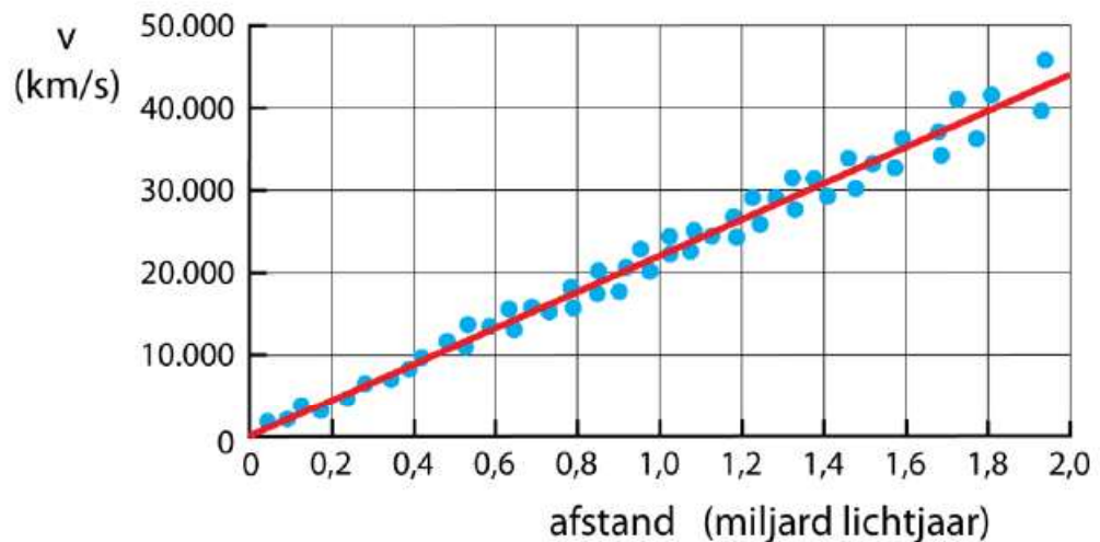
Figuur 76 Hubble diagram.
