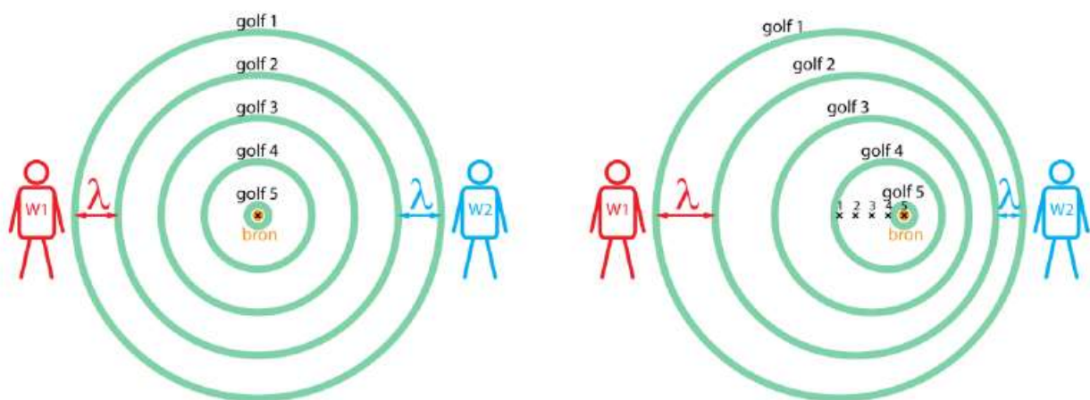
Figuur 62 Het dopplereffect. Links staat de bron stil. Rechts beweegt de bron van waarnemer W1 vandaan en naar waarnemer W2 toe. Waarnemer W1 ziet een grotere golflengte en W2 een kleinere golflengte. Voor W1 verschuift het spectrum naar het rood en voor W2 naar het blauw.
