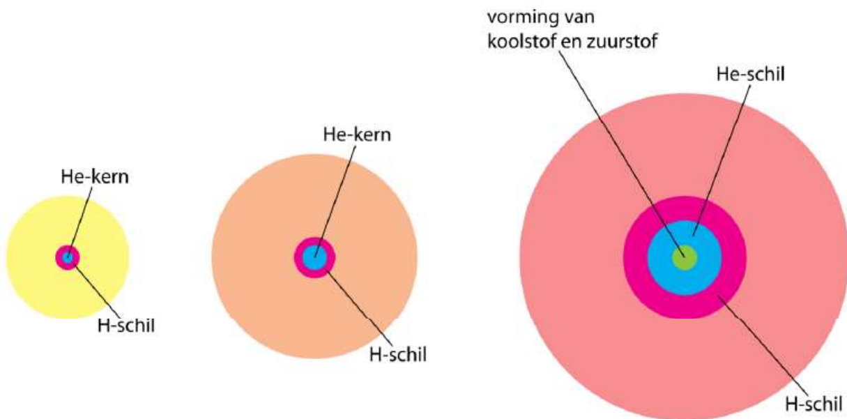
Figuur 69 De zon wordt een rode reus.
