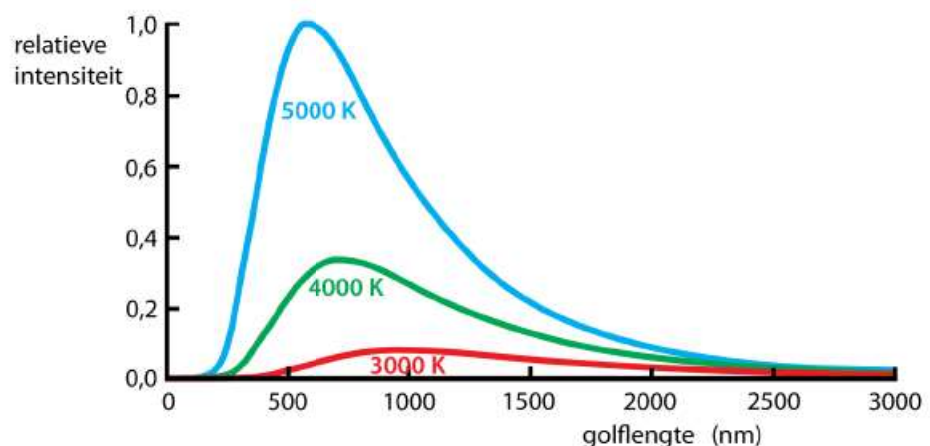
Figuur 50 Elektromagnetische straling. Naarmate de temperatuur toeneemt, wordt de hoeveelheid straling groter en schuift het de uitgezonden kleur van rood naar blauw.
