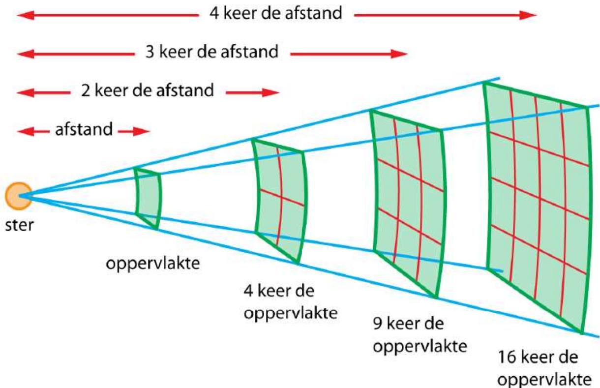
Figuur 51 De omgekeerde kwadratenwet. Als de afstand x -keer groter wordt neemt de intensiteit met 1/x^2 af.
