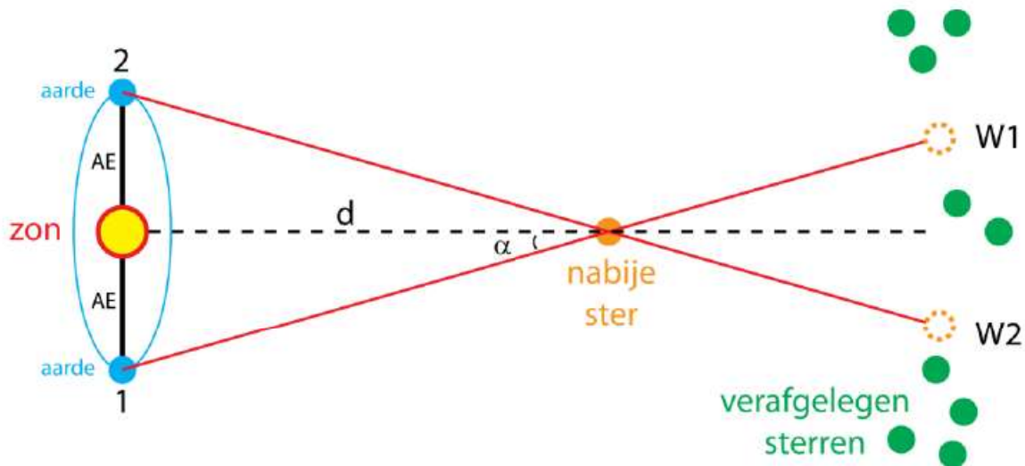
Figuur 48 De afstand van een nabije ster meten met behulp van parallax.
