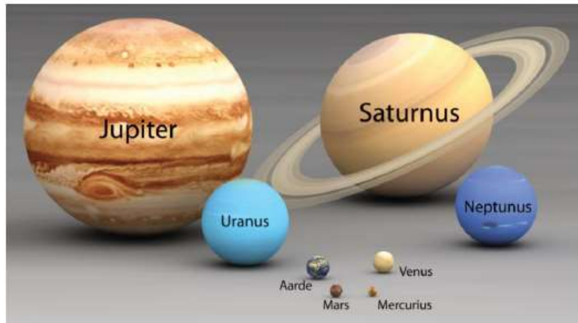
Figuur 12 Relatieve groottes van de planeten.
