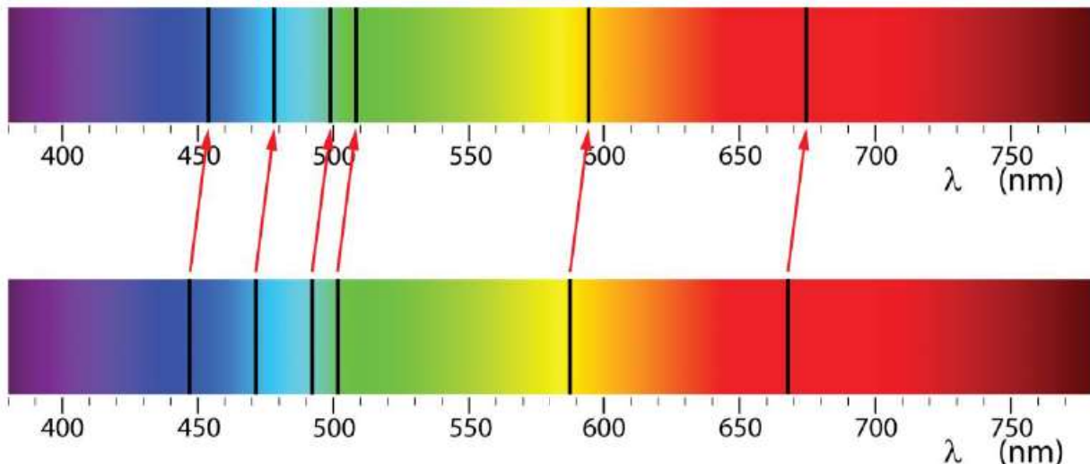
Figuur 63 Onderaan is het absorptiespectrum van helium. Van een ster wordt het bovenste spectrum waargenomen. De absorptielijnen zijn naar rood verschoven omdat de ster met grote snelheid van de aarde af beweegt. Helium heeft sterke absorptielijnen bij de volgende golflengten: 447,1 – 471,3 – 492,2 – 501,6 – 587,6 – 667,8 nm
