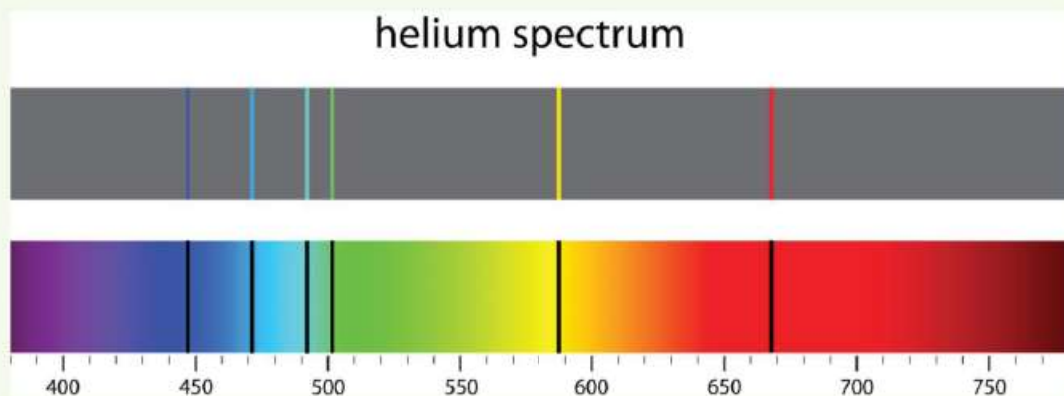
Figuur 59 Emissie- en absorptiespectrum van helium.
