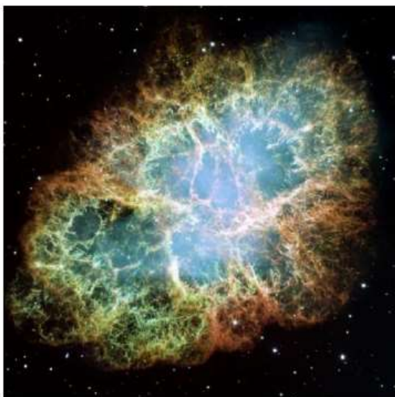
Figuur 24 Nevels in de Melkweg. Links: Krabnevel, rechts: Paardekopnevel.
