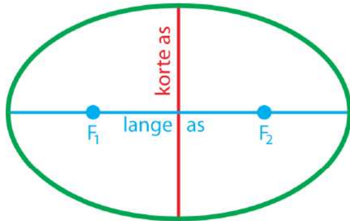
Figuur 39 Kepler's 3 e wet legt het verband tussen de lengte van de helft van de lange as en de omlooptijd.
