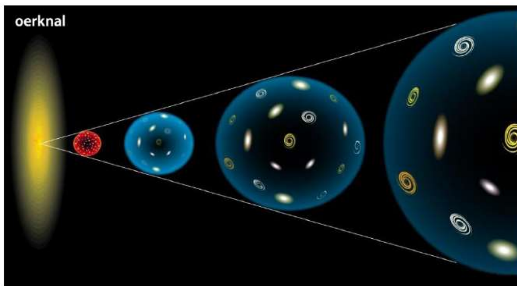
Figuur 75 Het heelal is 13,8 miljard jaar geleden ontstaan in één punt en is daarna steeds groter geworden.
