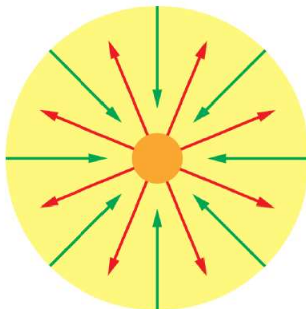
Figuur 68 Evenwicht in een ster. De rode pijlen geven de thermische druk weer. De groene pijlen geven de druk aan die door de gravitatiekracht wordt veroorzaakt.
