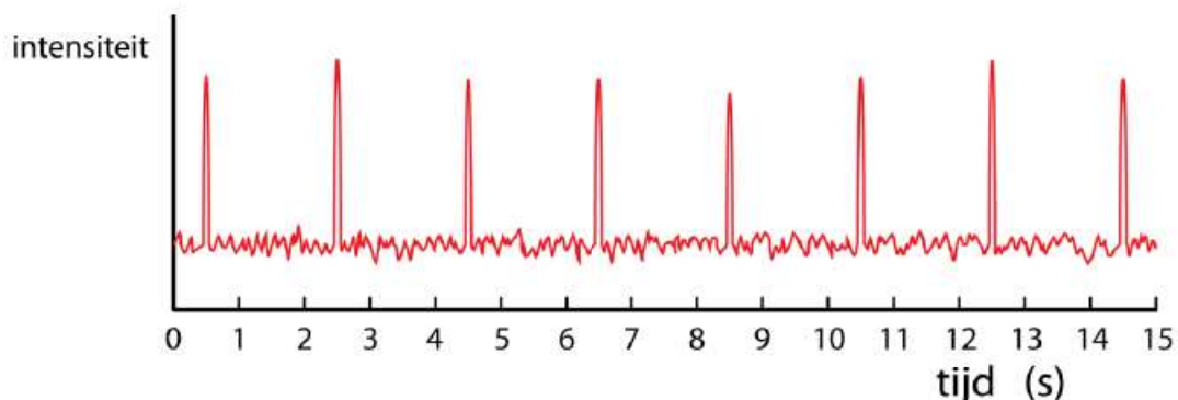
Figuur 72 Pieken elektromagnetische straling afkomstig van een pulsar.
