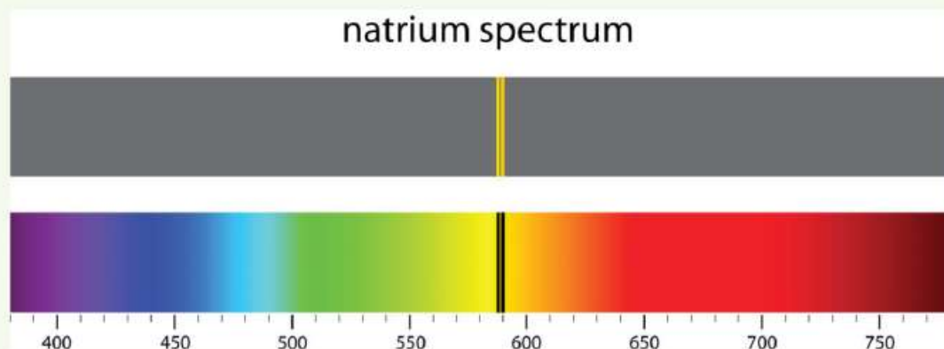
Figuur 57 Emissie- en absorptiespectrum van natrium.
