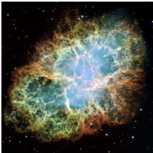
Figuur 74 Links: de Krabnevel, het restant van de supernova uit 1054. Rechts: het restant van de supernova uit 1572.
