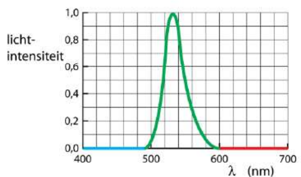
Figuur 56 Emissiespectrum. Groen licht wordt uitgestraald. Blauw en rood licht worden niet uitgestraald.
