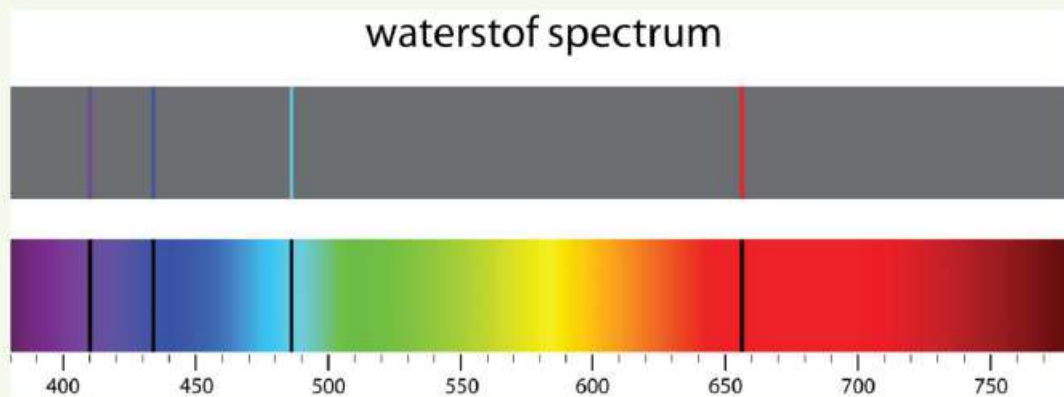
Figuur 58 Emissie- en absorptiespectrum van waterstof.
