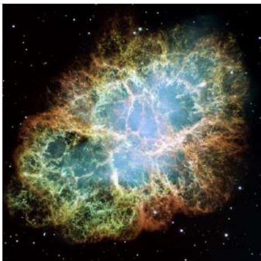
Figuur 76 Links: de Krabnevel, het restant van de supernova uit 1054. Rechts: het restant van de supernova uit 1572.
