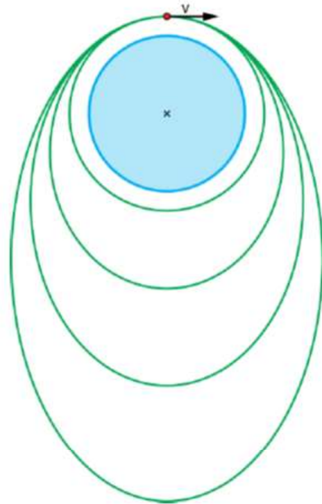
Figuur 32 Horizontaal weggeschoten projectiel met v_{\text{begin}} > 8,0 km/s.
