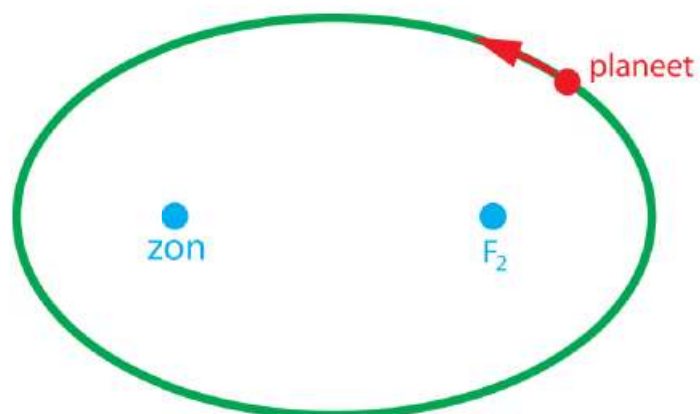
Figuur 34 Kepler's 1 e wet stelt dat planeten in ellipsvormige banen om de zon bewegen.
