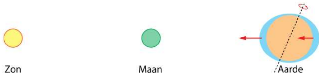
Figuur 10 Springtij bij nieuwe maan.
