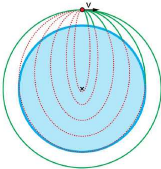
Figuur 31 Horizontaal weggeschoten projectiel met v_{\text{begin}} < 8,0 km/s.
