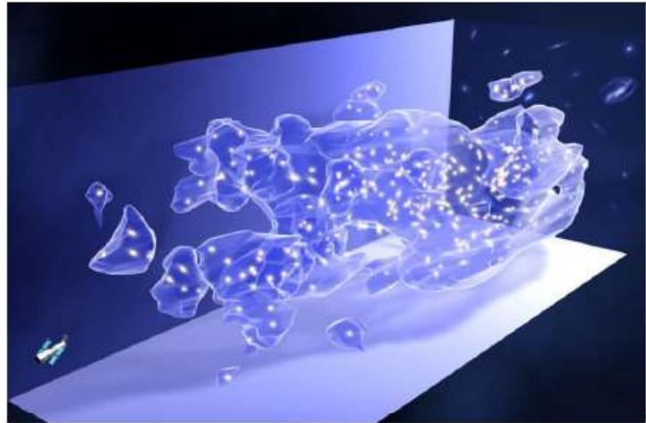
Figuur 86 De kromming van de ruimte in kaart gebracht via gravitatielenzen.
