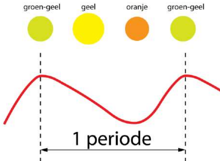
Figuur 58 Periodieke variatie in lichtsterkte en kleur van een Cepheïde ster.
