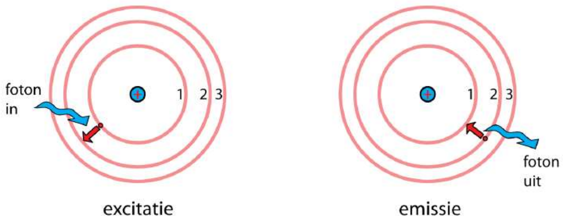
Figuur 42 Excitatie: een atoom neemt een foton op. Emissie: een atoom zendt een foton uit.
