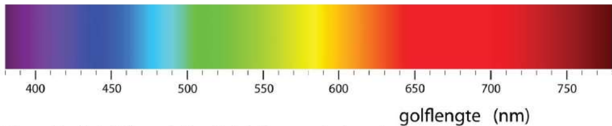
Figuur 41 Het zichtbare deel van het elektromagnetisch spectrum.
