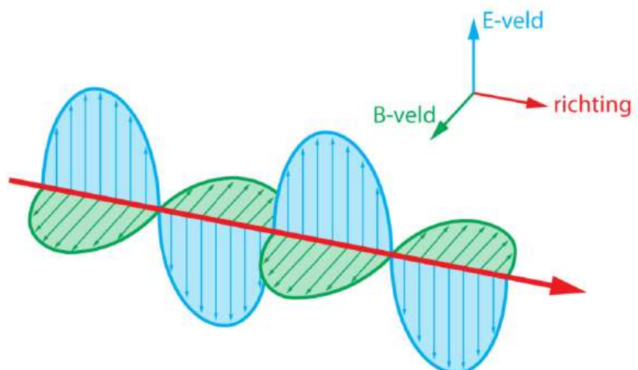
Figuur 39 Elektromagnetische golf.
