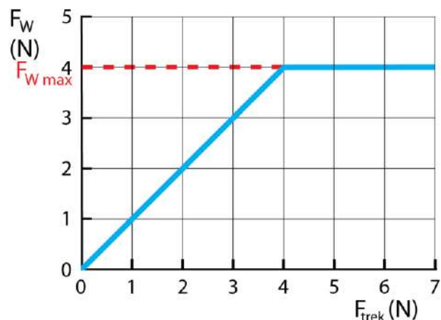
Figuur 36 Om twee ruwe oppervlakken over elkaar heen te schuiven is een kracht nodig. Als F_{\text{trek}} de kleiner is dan F_{W \text{ max}} komt het voorwerp niet in beweging.
