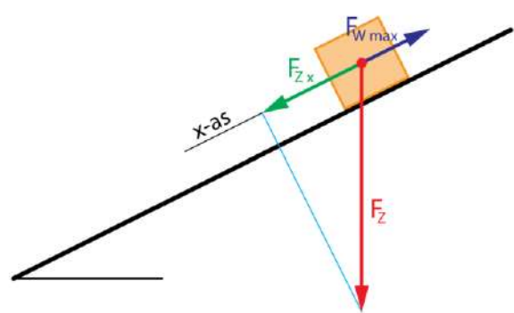
Figuur 42 Blok versnelt naar beneden. Versnellen \rightarrow F_{Zx} - F_{W \text{ max}} = m \cdot a .
