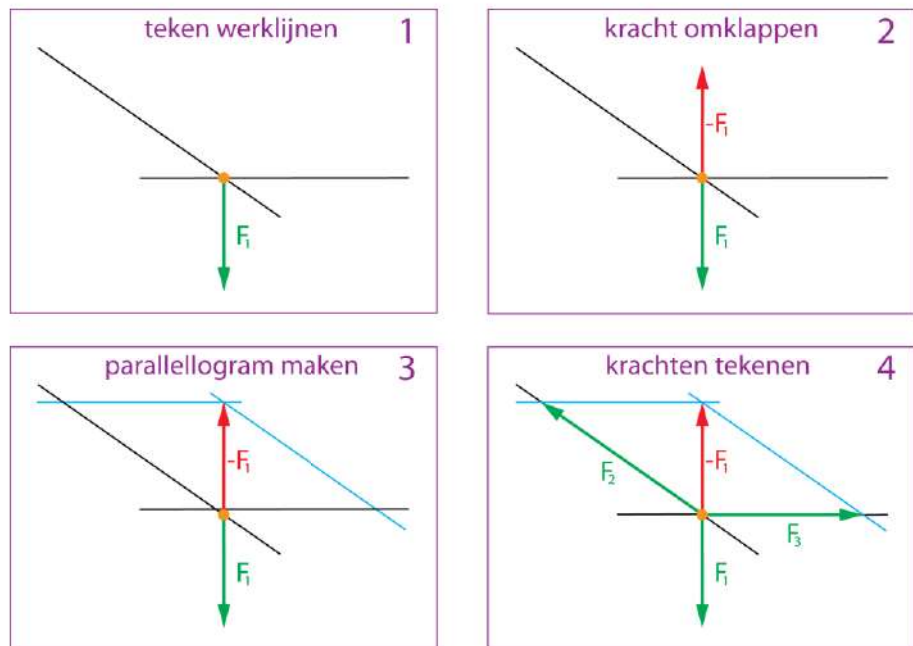
Figuur 10 Bepaal de krachten F_2 en F_3 zodat F_1 + F_2 + F_3 = 0 .
