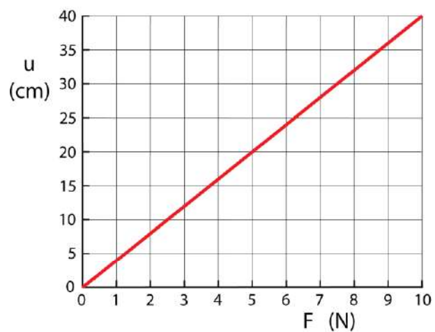
Figuur 19 ( u , F )-diagram van een spiraalveer.
