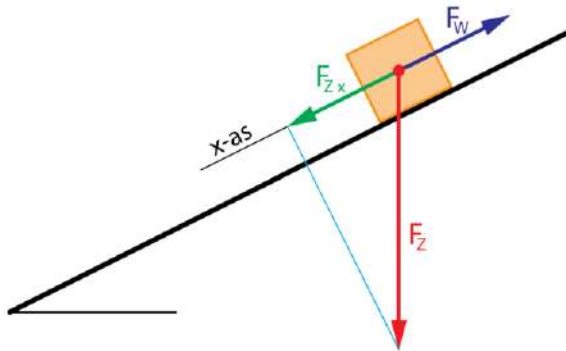
Figuur 41 Blok staat stil op een helling. Stilstaan \rightarrow F_{Zx} = F_W .
