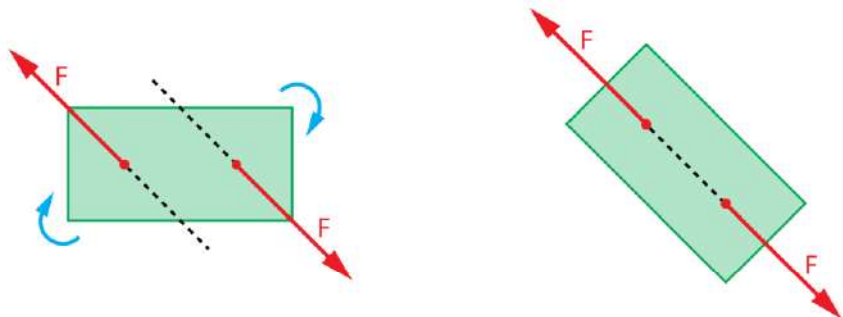
Figuur 24 Links: op een blok werken twee krachten waarbij de werklijnen elkaar niet snijden. Het blok zal hierdoor gaan draaien. Rechts: het draaien stopt als de werklijnen elkaar snijden of samenvallen.
