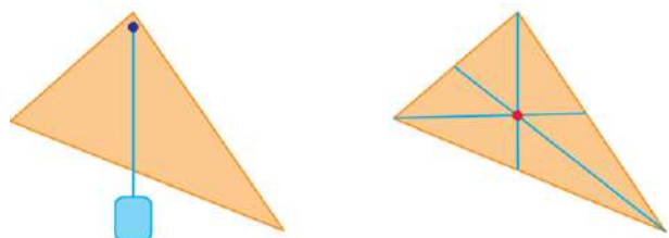
Figuur 14 Methode om het zwaartepunt te bepalen.
