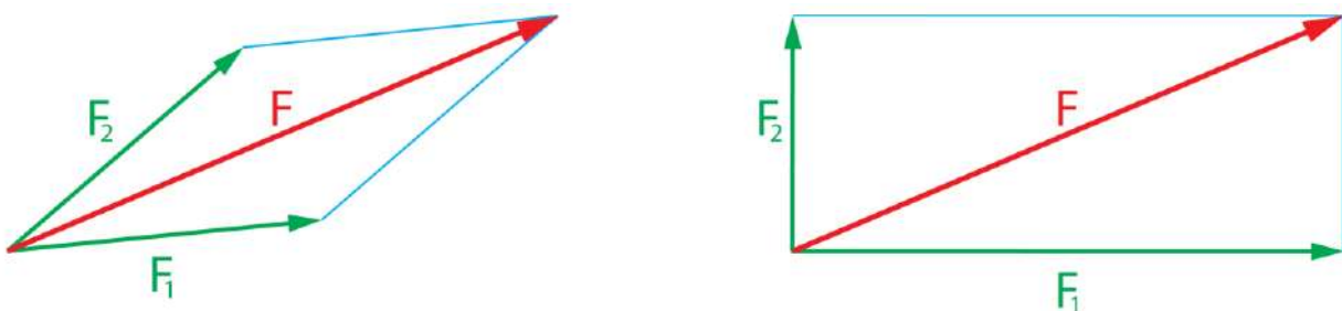
Figuur 7 Links is kracht F gesplitst in componenten F_1 en F_2 die niet loodrecht op elkaar staan. Recht is dezelfde kracht gesplitst in F_1 en F_2 die wel loodrecht op elkaar staan.
