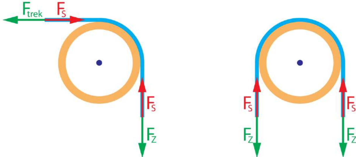
Figuur 23 Als het uitgerekte koord een bocht maakt, bijvoorbeeld doordat het om een wiel is gelegd, zal de spankracht de bocht omgaan.
