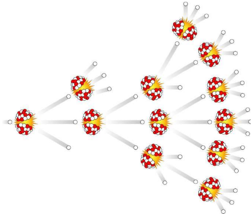
Figuur 35 Splijting van een U-235 kern.
