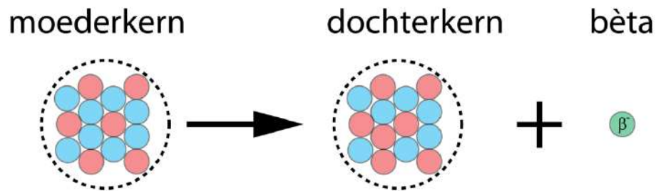
Figuur 7 \beta^- -verval van C-14. blauw = proton wit = neutron
