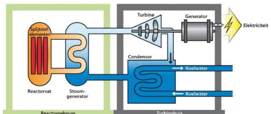
Figuur 38 De werking van een kerncentrale.
