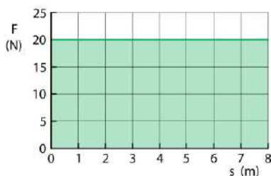
Figuur 5 De arbeid die F verricht is gelijk aan de oppervlakte onder de (F, s)-grafiek.
