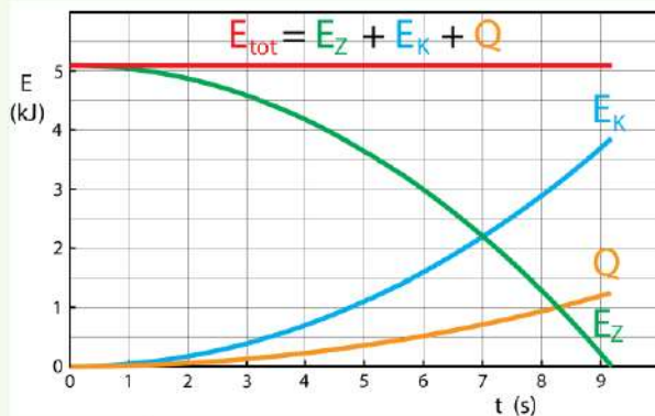
Figuur 21 (E, t)-diagram van de skater.
