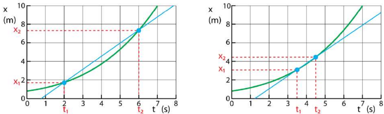
Figuur 16 De gemiddelde snelheid tussen t_1 en t_2 . Links liggen t_1 en t_2 ver uit elkaar en rechts liggen ze vlak naast elkaar.
