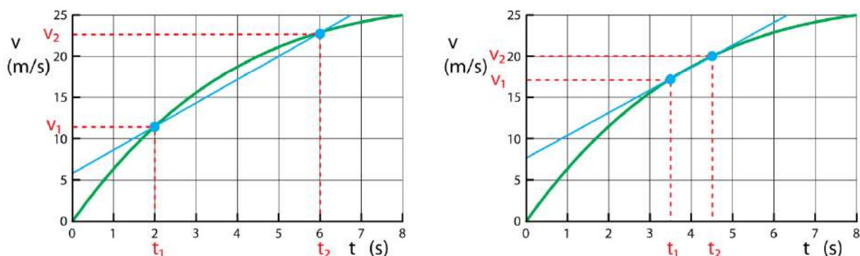
Figuur 24 De gemiddelde versnelling tussen t_1 en t_2 . Links liggen t_1 en t_2 ver uit elkaar en rechts liggen ze vlak naast elkaar.
