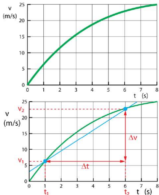
Figuur 23 De gemiddelde versnelling bepalen tussen t_1 en t_2 .
