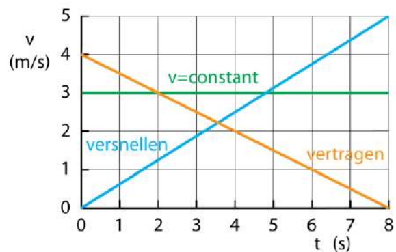
Figuur 18 (v, t)-diagram.
