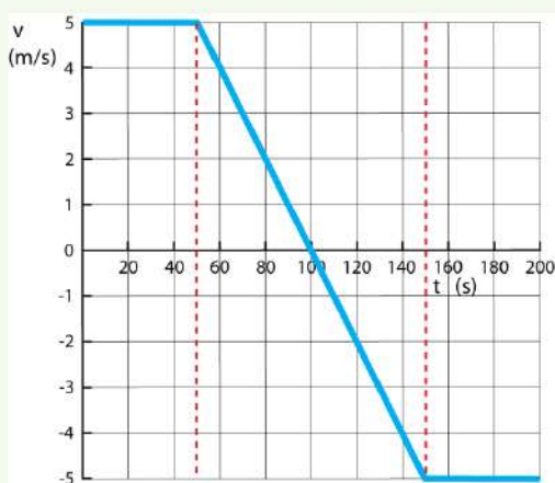
Figuur 36 Links (v, t)-diagram, rechts (x, t)-diagram.
