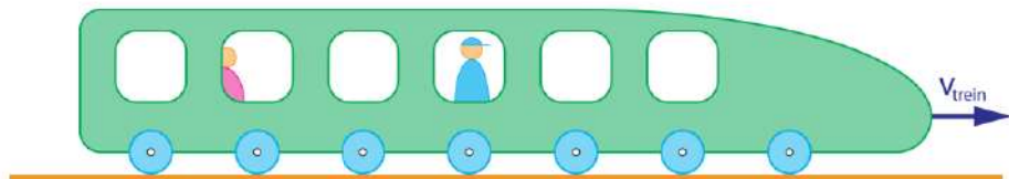
Figuur 12 Snelheden optellen.
