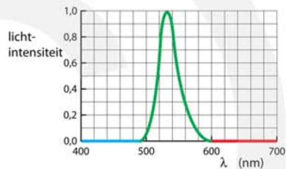
Figuur 56 Emissiespectrum. Groen licht wordt uitgestraald. Blauw en rood licht worden niet uitgestraald.
