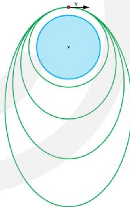
Figuur 33 Horizontaal weggeschoten projectiel met v_{\text{begin}} > 8,0 km/s.
