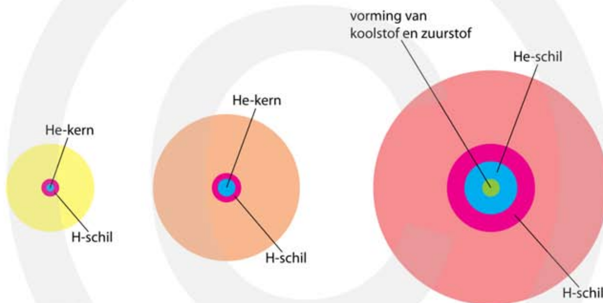
Figuur 69 De zon wordt een rode reus.
