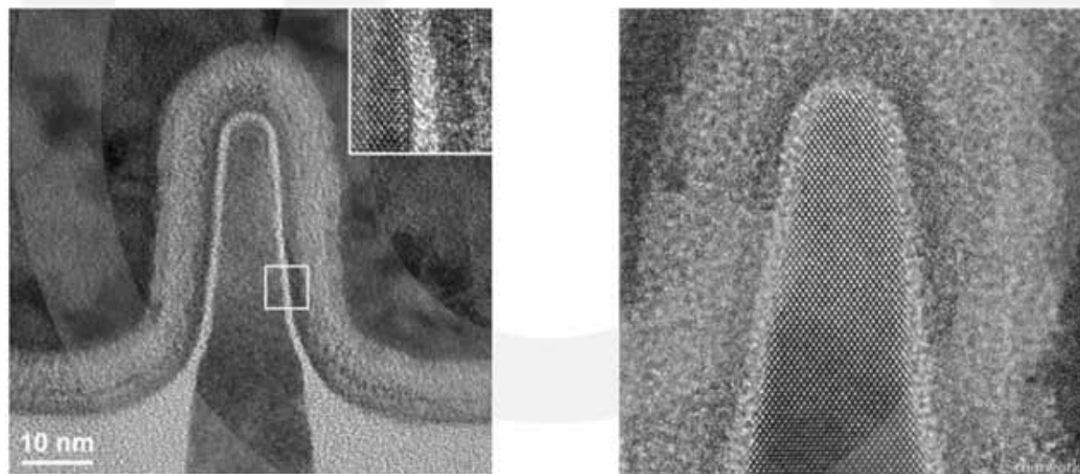
Figuur 4 HR-TEM beeld van een 22 nm 3D transistor die momenteel worden ontwikkeld. Bij de vergroting zie je siliciumatomen. Bij de vervaardiging wordt extreme UV-straling (EUV) met een golflengte tussen 5 en 10 nm gebruikt.
