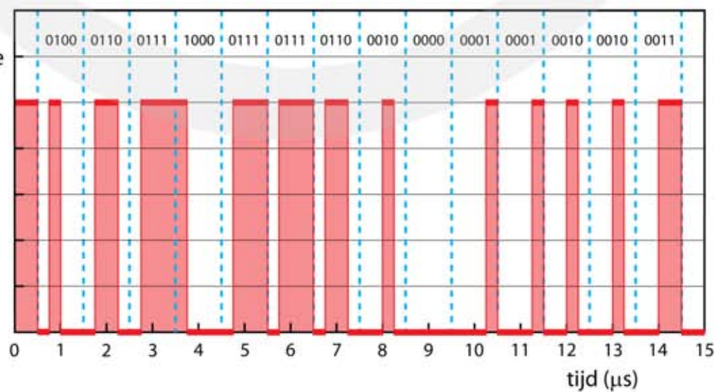
Figuur 27 Een binaire code wordt uitgezonden door EM-straling met amplitudemodulatie.
