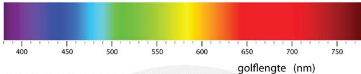
Figuur 11 Zichtbare deel van het elektromagnetisch spectrum.
