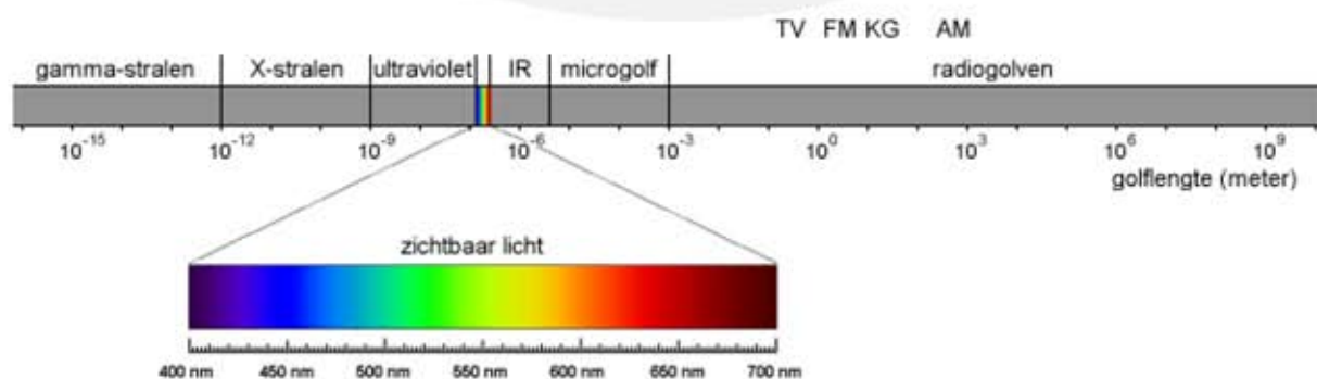
Figuur 12 Elektromagnetische straling.
