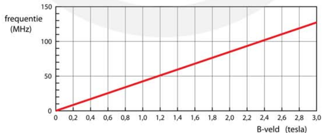
Figuur 43 Er is een recht evenredig verband tussen de magnetische veldsterkte en de frequentie van de EM-straling waarbij de oriëntatie van de protonspins omkeert.
