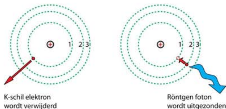
Figuur 34 Scherpe pieken in het röntgenspectrum ontstaan doordat een elektron uit de L-schil naar een vrijgekomen plaats in de K-schil springt en daarbij een röntgenfoton uitzendt.
