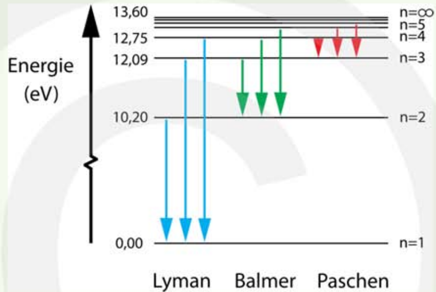
Figuur 18 Vereenvoudigd energieniveauschema voor waterstof.
