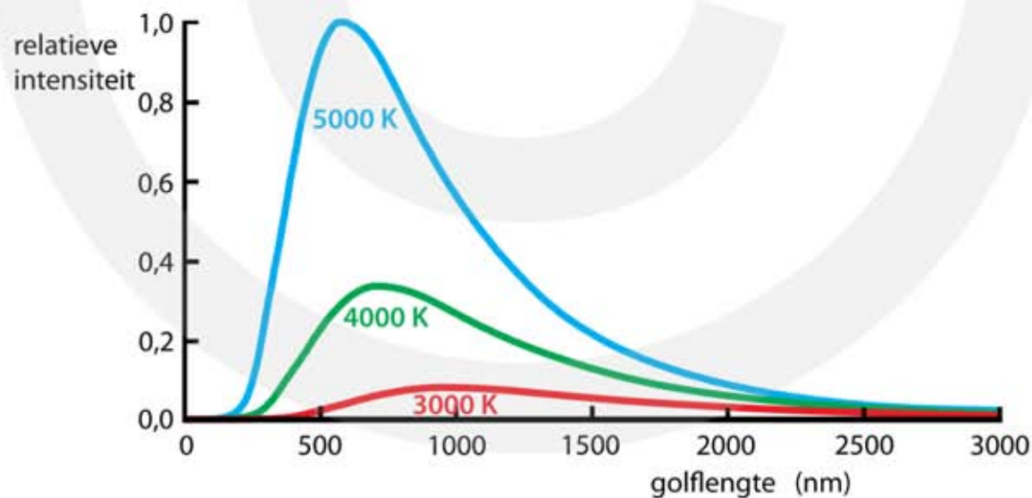
Figuur 13 Ieder voorwerp zendt EM-straling uit. Als de temperatuur toeneemt wordt er meer straling uitgezonden en verschuift het maximum van de grafiek naar een kleinere golflengte.
