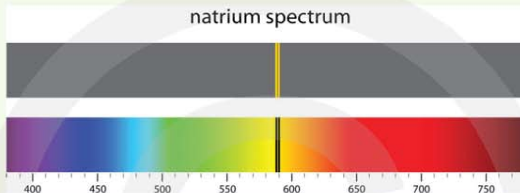
Figuur 20 Emissie- en absorptiespectrum van natrium.
