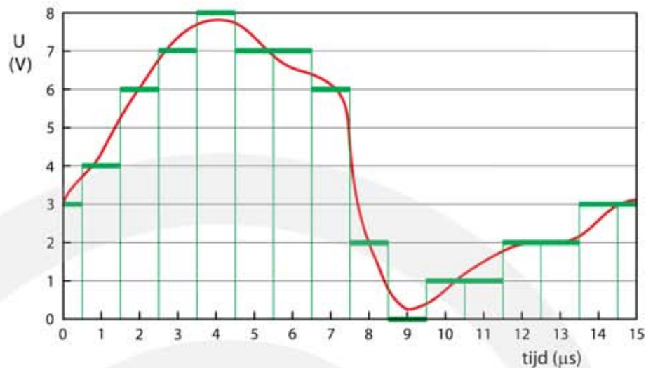
Figuur 28 Digitale communicatie. Een binaire code wordt zonder storing ontvangen en omgezet in een spanning. Er is een afwijking tussen het oorspronkelijke signaal (rood) en het overgebrachte signaal (groen).
