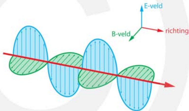
Figuur 10 Trillingen in het elektrisch veld (E-veld) en magnetisch veld (B-veld) verspreiden zich samen als elektromagnetische golf met een vaste snelheid door de ruimte.
