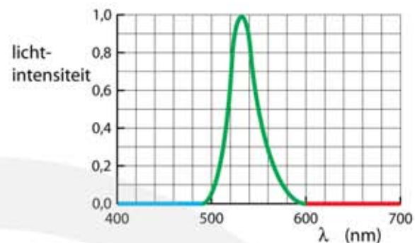
Figuur 16 Emissiespectrum. Groen licht wordt uitgestraald. Blauw en rood licht worden niet uitgestraald.
