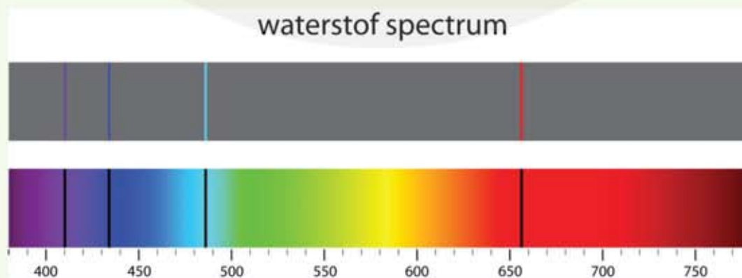
Figuur 19 Emissie- en absorptiespectrum van waterstof.
