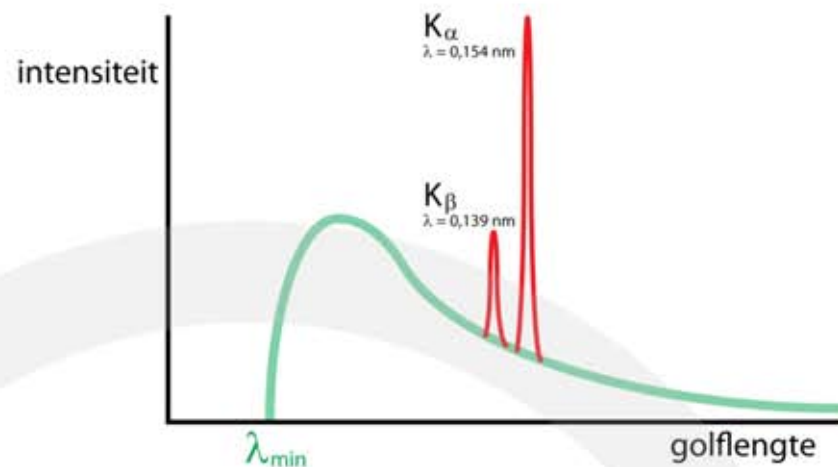
Figuur 33 Het spectrum van röntgenstralen opgewekt in een anode van koper.
