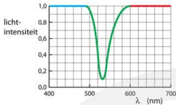
Figuur 15 Absorptiespectrum. Groen licht wordt geabsorbeerd. Blauw en rood licht worden doorgelaten.
