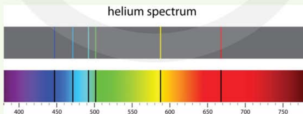
Figuur 21 Emissie- en absorptiespectrum van helium.
