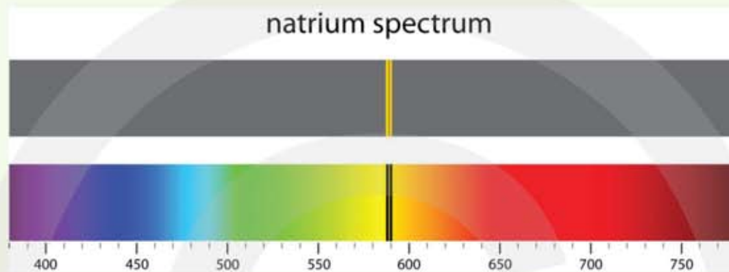
Figuur 46 Emissie- en absorptiespectrum van natrium.
