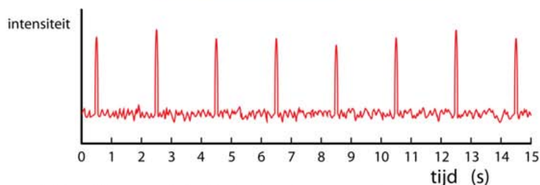
Figuur 74 Pieken elektromagnetische straling afkomstig van een pulsar.
