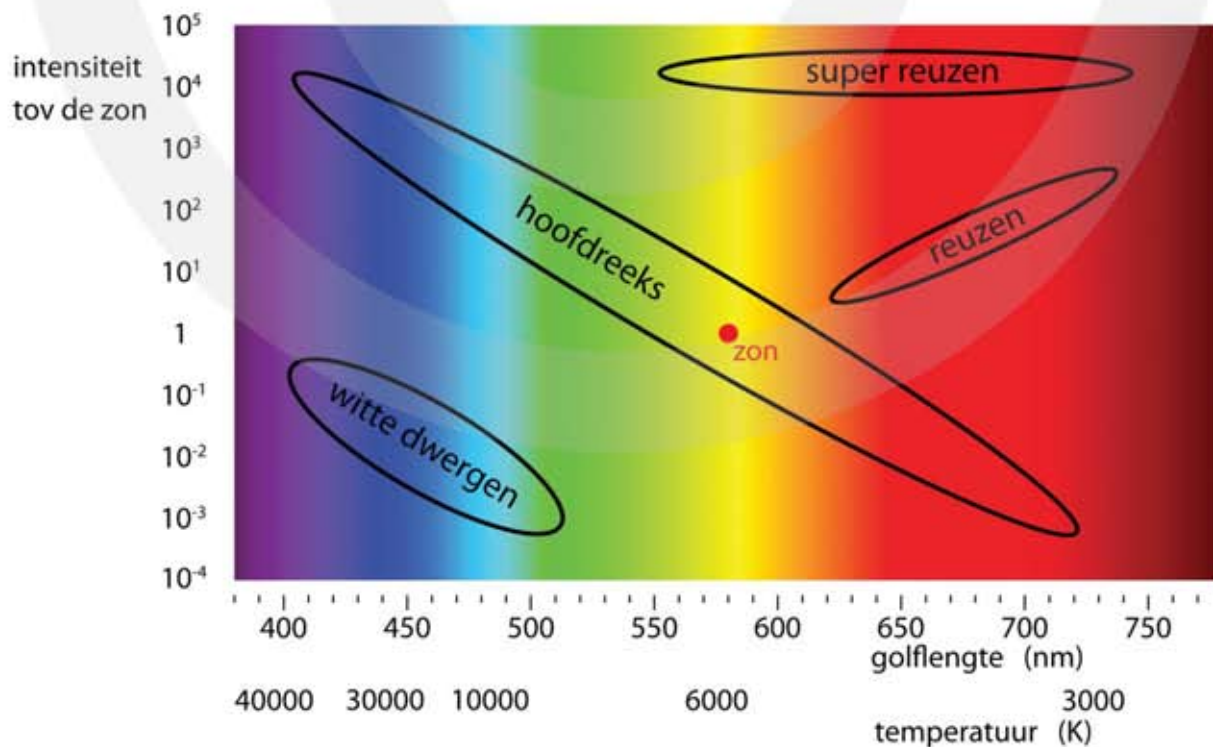
Figuur 61 Hertzsprung-Russell diagram. Op de horizontale as staat de golflengte die het meest wordt uitgestraald en daaronder de bijbehorende oppervlaktetemperatuur. Op de verticale as staat de intensiteit ten opzichte van de intensiteit van de zon.
