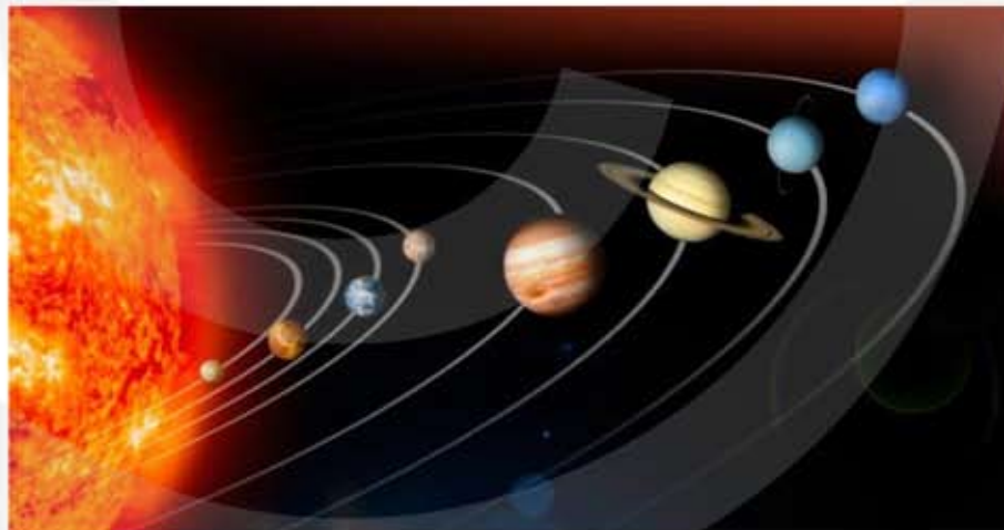
Figuur 11 Het zonnestelsel. De afstanden zijn niet op schaal.
