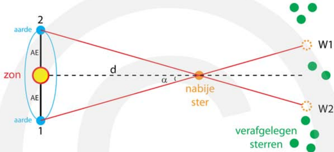
Figuur 57 De afstand van een nabije ster meten met behulp van parallax.
