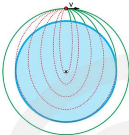
Figuur 31 Horizontaal weggeschoten projectiel met v_{\text{begin}} < 8,0 \text{ km/s} .
