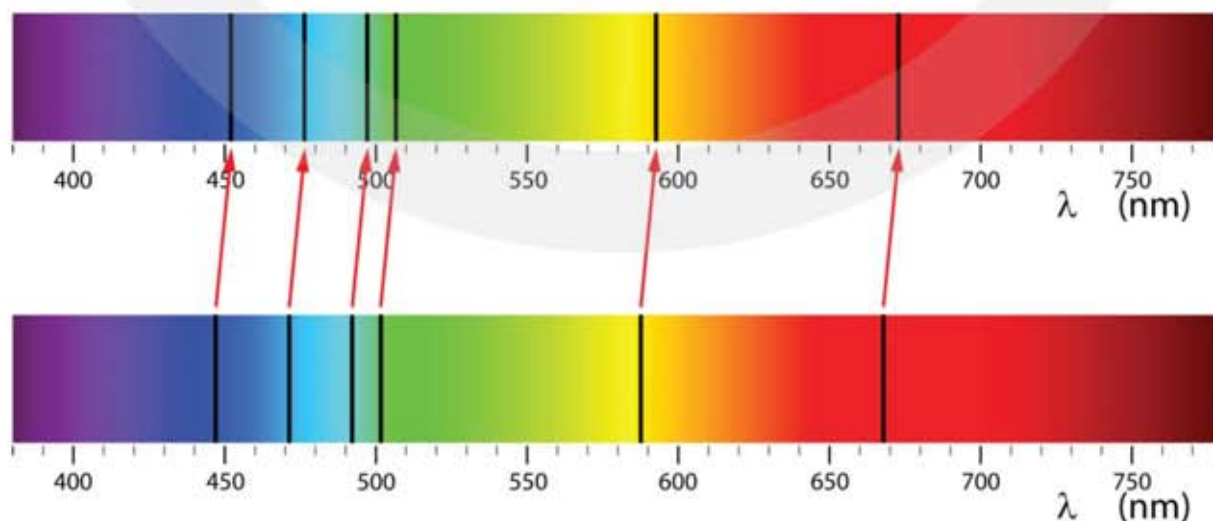
Figuur 65 Onderaan is het absorptiespectrum van helium. Van een ster wordt het bovenste spectrum waargenomen. De absorptielijnen zijn naar rood verschoven omdat de ster met grote snelheid van de aarde af beweegt. Helium heeft sterke absorptielijnen bij de volgende golflengten: 447,1 – 471,3 – 492,2 – 501,6 – 587,6 – 667,8 nm
