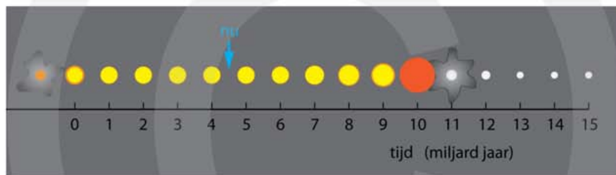
Figuur 66 De levensloop van de zon.
