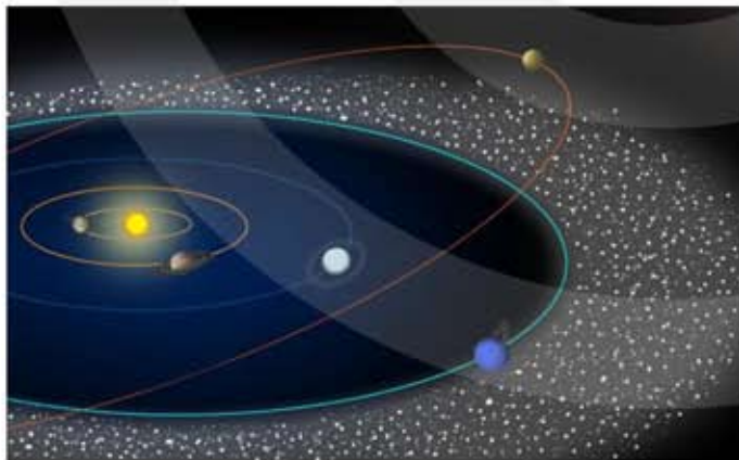
Figuur 13 De Kuipergordel met dwergplaneet Pluto.
