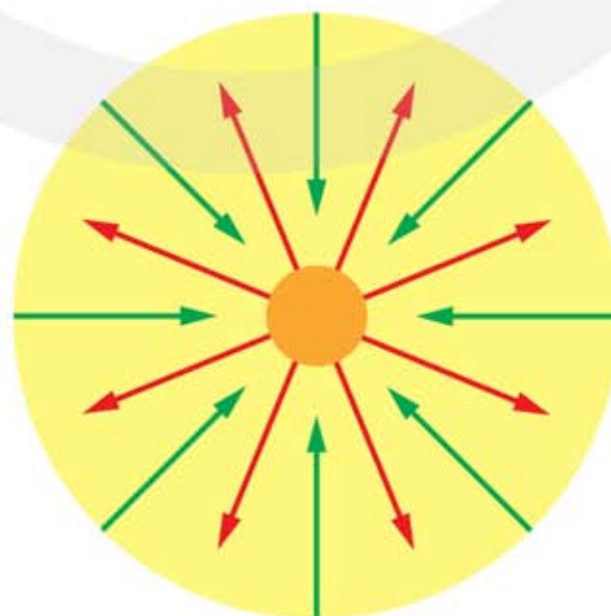
Figuur 70 Evenwicht in een ster. De rode pijlen geven de thermische druk weer. De groene pijlen geven de druk aan die door de gravitatiekracht wordt veroorzaakt.
