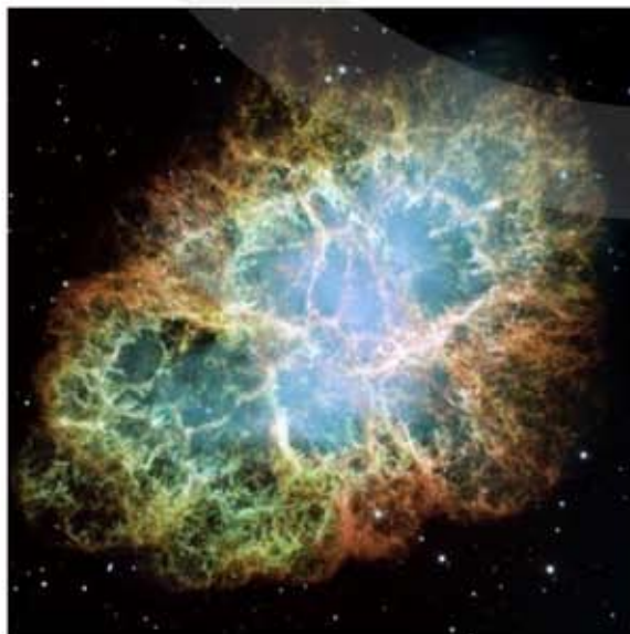
Figuur 24 Nevels in de Melkweg. Links de Krabnevel en rechts de Paardekopnevel.
