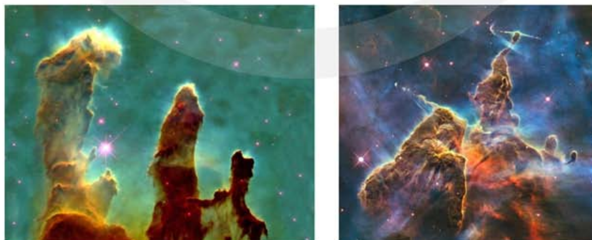
Figuur 67 In een stervormende nevel is 4,6 miljard jaar geleden de zon ontstaan. Links: stervorming in de Eagle nevel ; Rechts: stervorming in de Carina nevel.
