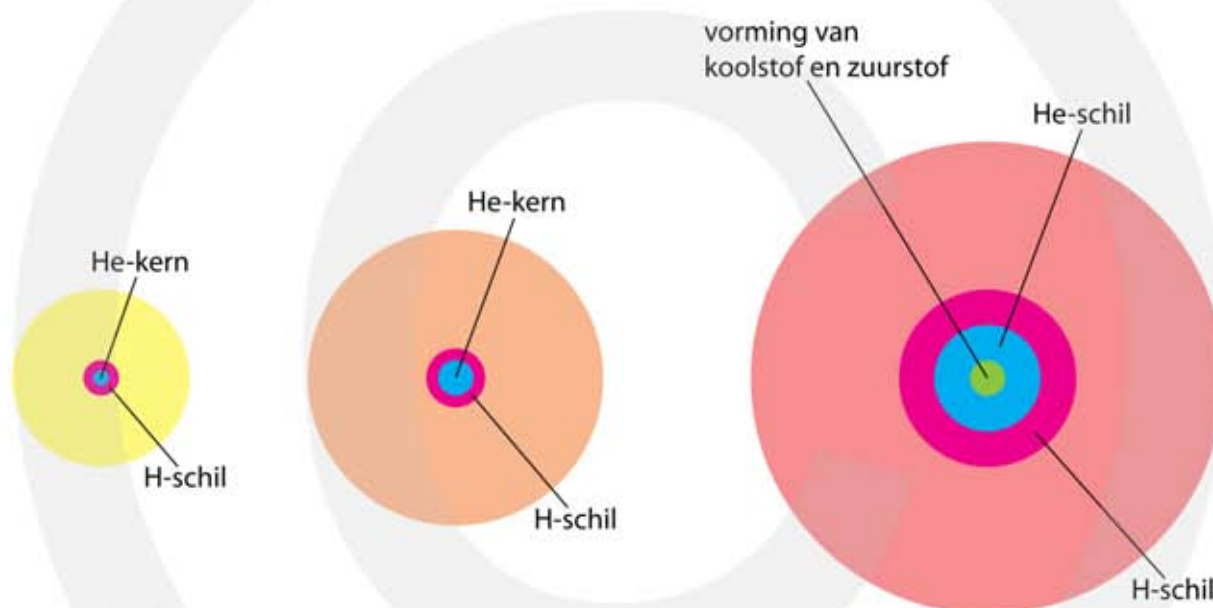
Figuur 71 De zon wordt een rode reus.
