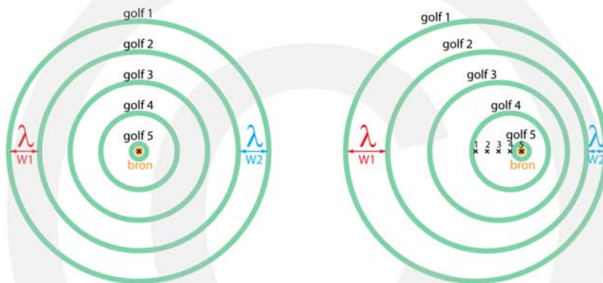
Figuur 64 Het doppler effect. Links staat de bron stil. Rechts beweegt de bron van waarnemer W1 vandaan en naar waarnemer W2 toe. Waarnemer W1 ziet een grotere golflengte en W2 een kleinere golflengte. Voor W1 verschuift het spectrum naar het rood en voor W2 naar het blauw.
