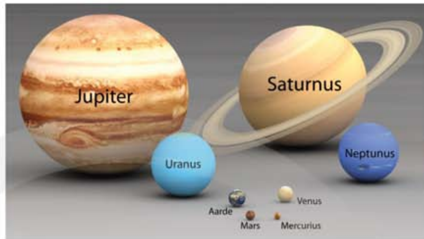
Figuur 12 Relatieve groottes van de planeten.
