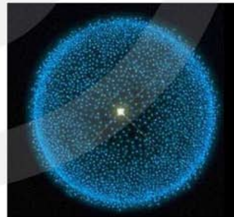
Figuur 14 De Oortwolk.
