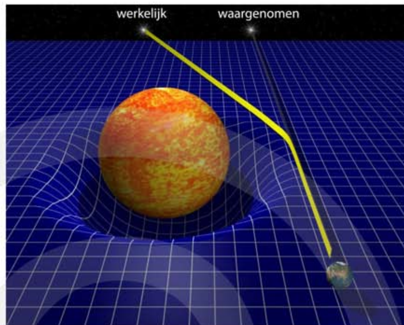
Figuur 81 Licht van een ster buigt om de zon heen. Hierdoor verandert de plaats van de ster aan de hemel.
