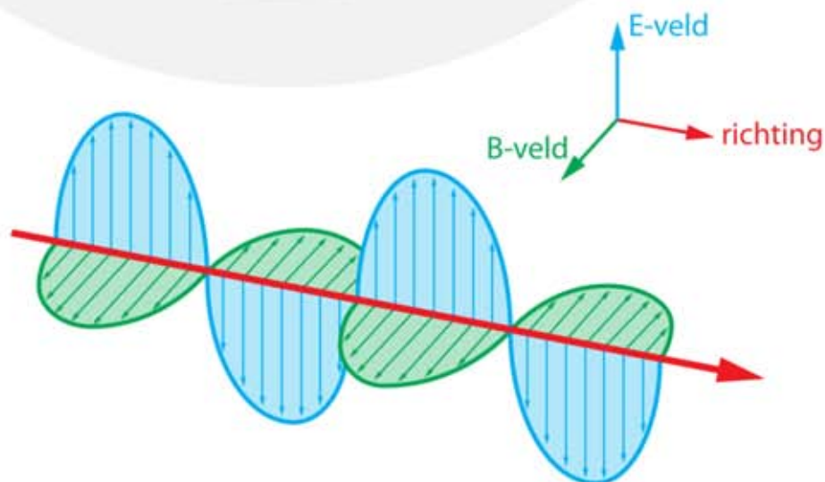
Figuur 39 Elektromagnetische golf.
