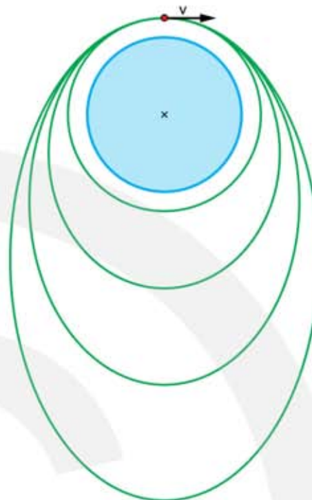
Figuur 32 Horizontaal weggeschoten projectiel met v_{\text{begin}} > 8,0 \text{ km/s} .
