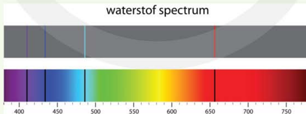
Figuur 47 Emissie- en absorptiespectrum van waterstof.
