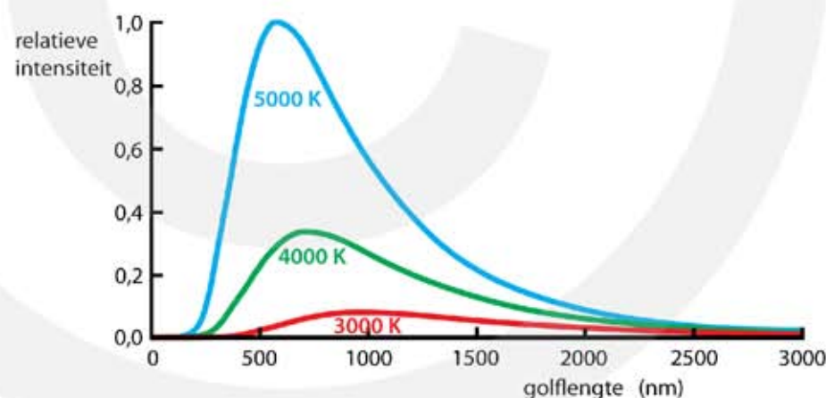
Figuur 59 Elektromagnetische straling. Naarmate de temperatuur toeneemt, wordt de hoeveelheid straling groter en schuift het de uitgezonden kleur van rood naar blauw.
