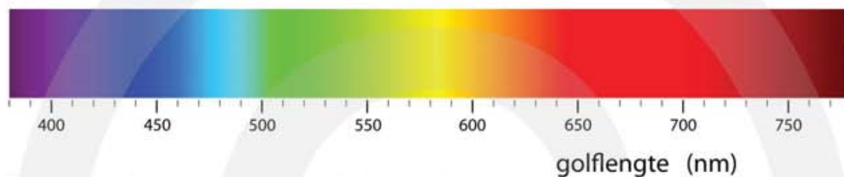
Figuur 41 Het zichtbare deel van het elektromagnetisch spectrum.
