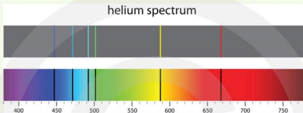
Figuur 48 Emissie- en absorptiespectrum van helium.
