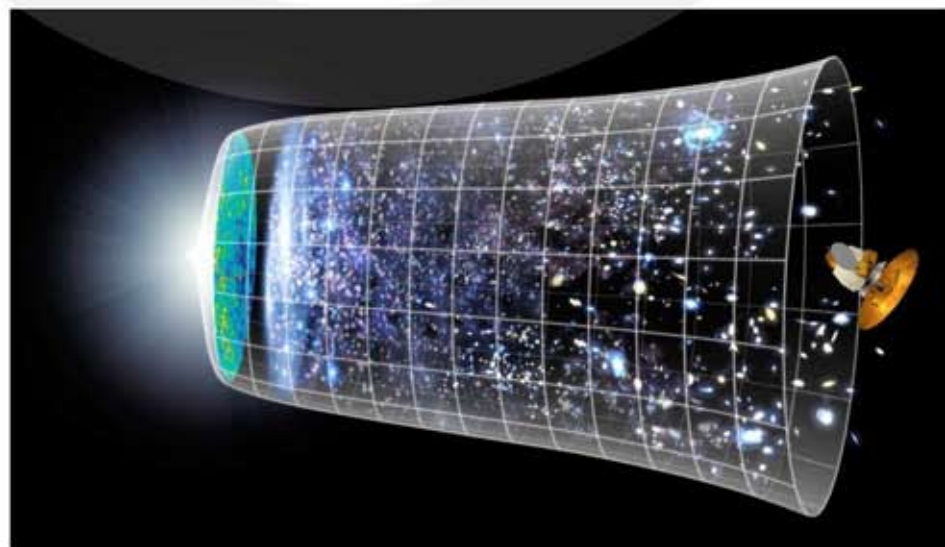
Figuur 92 De evolutie van het heelal vanaf de oerknal tot nu.
