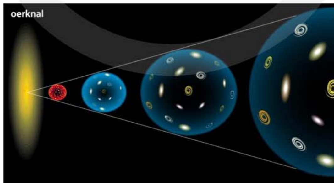
Figuur 77 Het heelal is 13,8 miljard jaar geleden ontstaan in één punt en is daarna steeds groter geworden.
