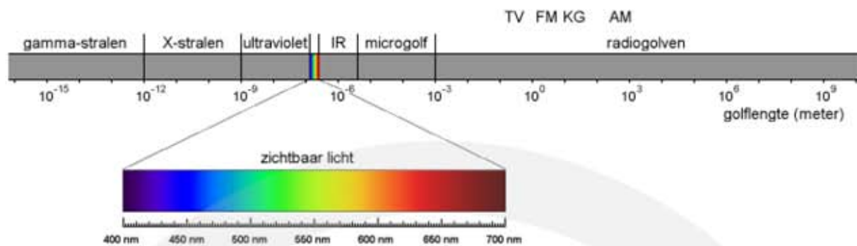
Figuur 40 Elektromagnetische straling.
