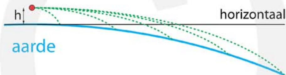
Figuur 27 Invloed van de kromming van de aarde op het vallen van een weggeschoten projectiel.
