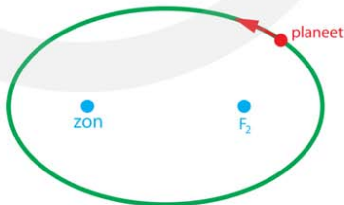
Figuur 34 Kepler's 1 e wet stelt dat planeten in ellipsvormige banen om de zon bewegen.
