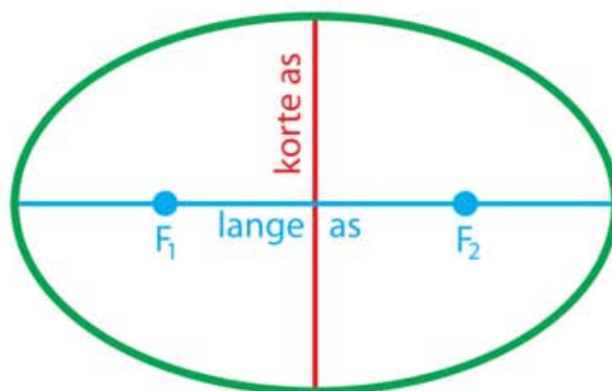
Figuur 36 Kepler's 3 e wet legt het verband tussen de lengte van de helft van de lange as en de omlooptijd.
