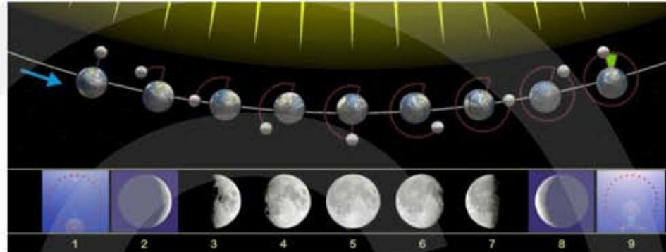
Figuur 6 De schijngestalten van de maan.
